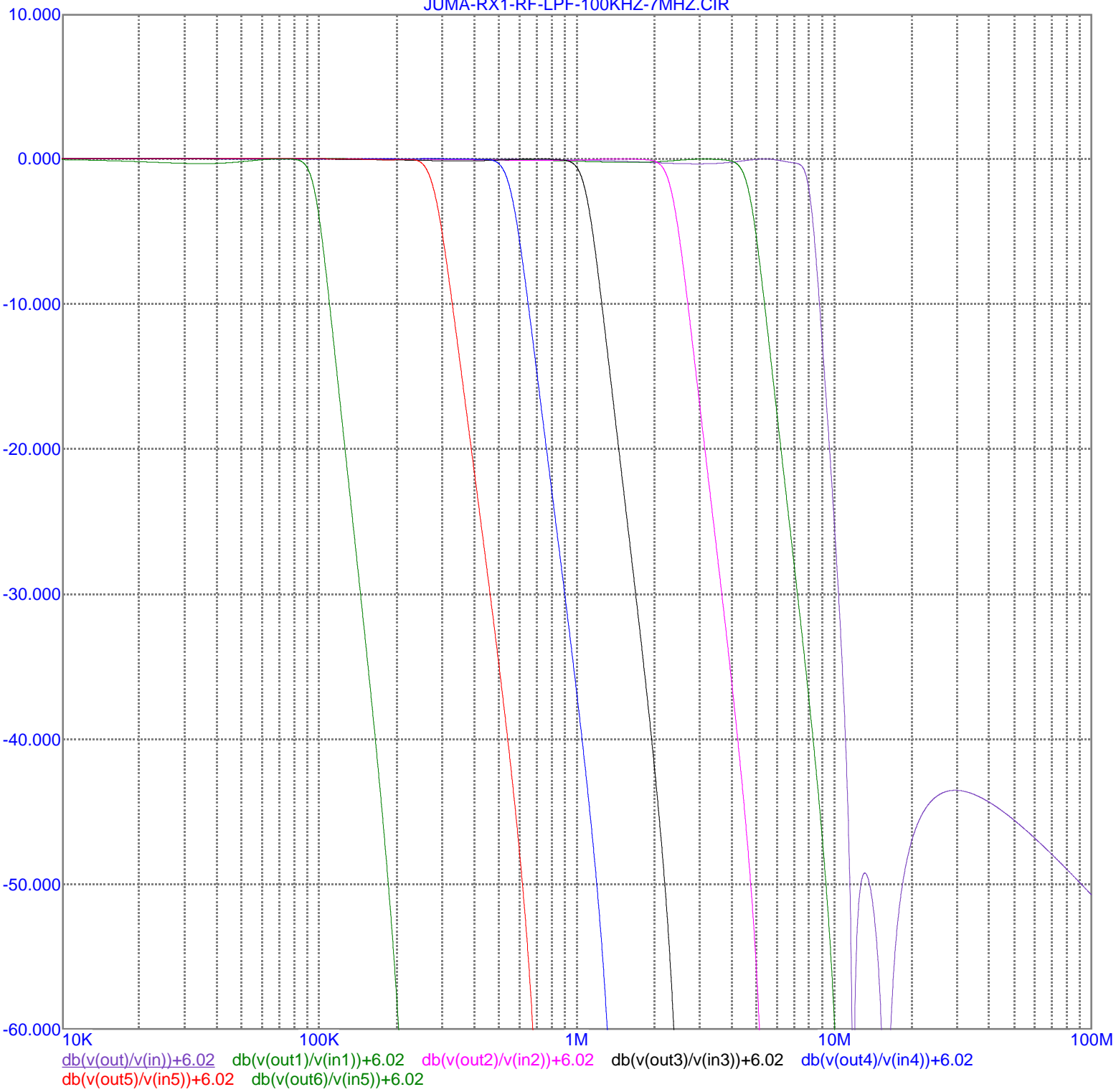
JUMA-RX1-RF-LPF-100KHZ-7MHZ.CIR
